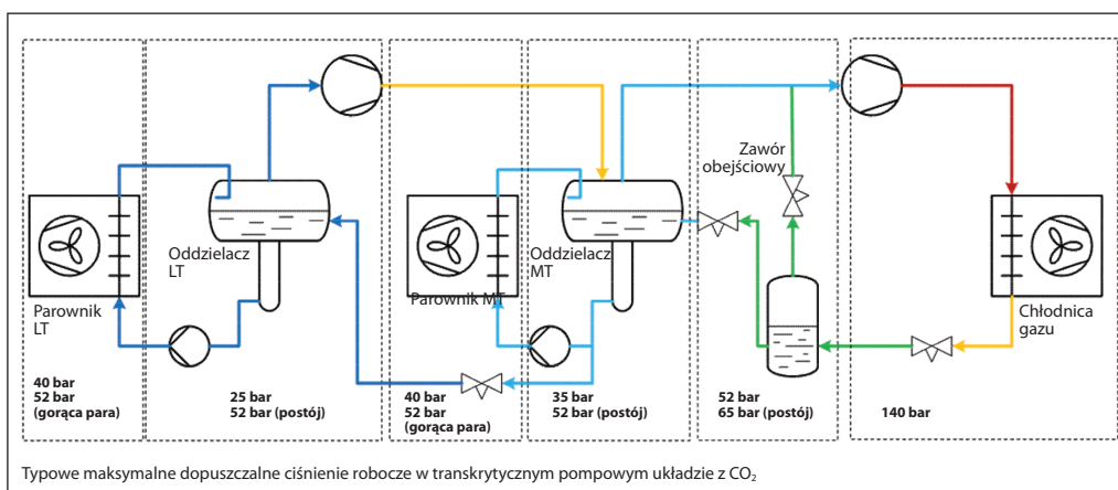
Rysunek 11.39: Typowe wartości maksymalnego dopuszczalnego ciśnienia roboczego w przemysłowym transkrytycznym układzie z CO 2 z zasilaniem pompowym
