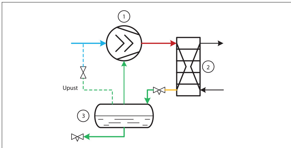
Rysunek 12.3.8: Ekonomizer bezprzeponowy z rurociągim upustowym
