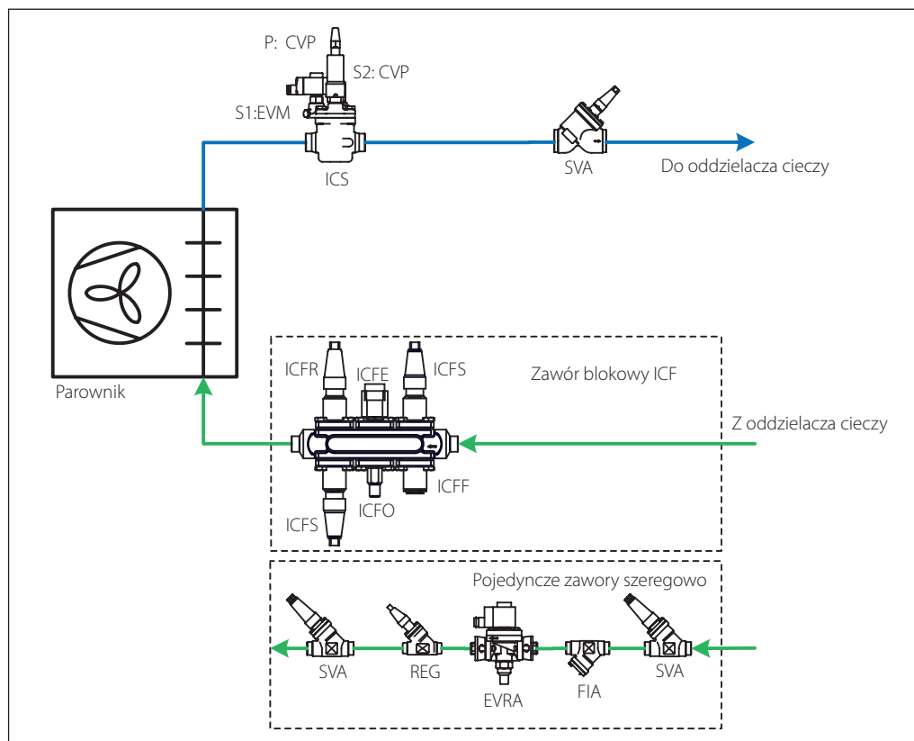
Przykład instalacji 5.1.2: Regulacja ciśnienia parowania dla dwóch alternatywnych nastaw
