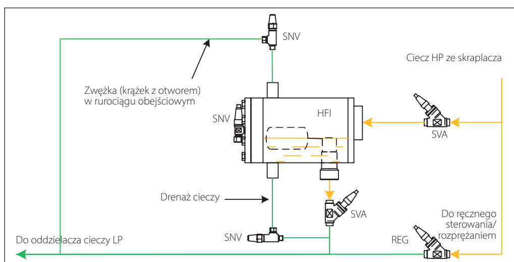
Przykład instalacji 4.1.6: Instalacja zaworu HFI z korpusem z dwoma dodatkowymi króćcami, z dala od skraplacza.
